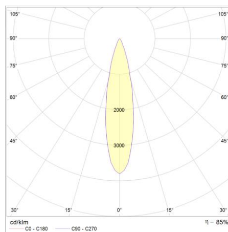
DIAGRAMMA POLARE 38°
