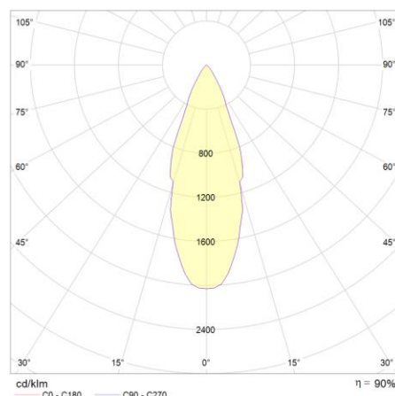
DIAGRAMMA POLARE 38°
