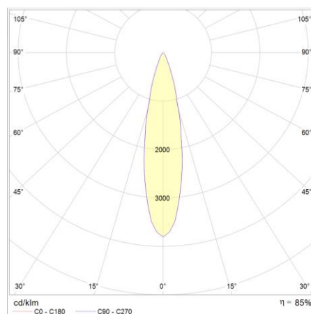
DIAGRAMMA POLARE 23°
