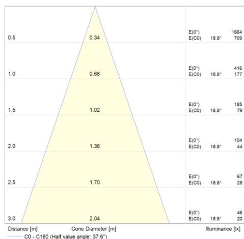
DIAGRAMMA CONICO 38°
